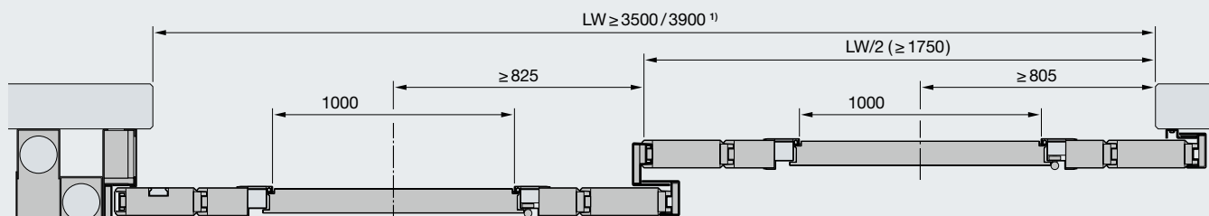
Parte del tirador Posibilidad de EI 2 30, EI 2 90 con puerta peatonal incorporada
