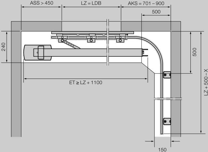
Guías ES (carril sencillo, automatismo montado en el techo B)
