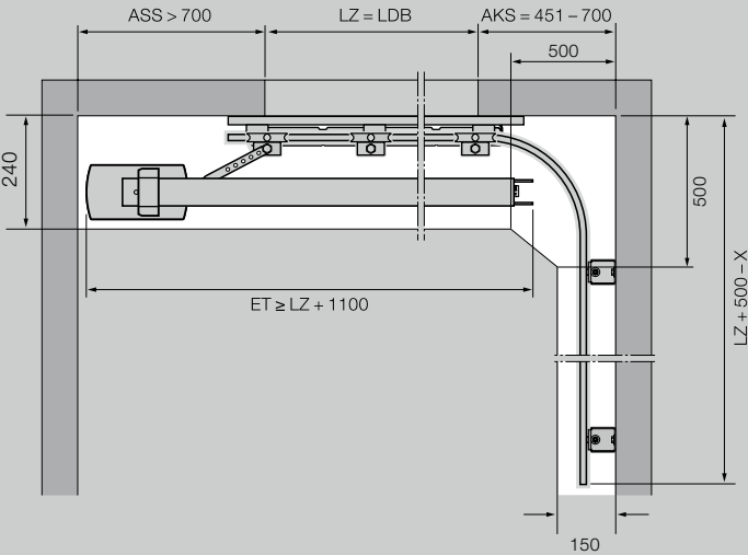
Guías DS (carril doble, automatismo montado en la pared)
